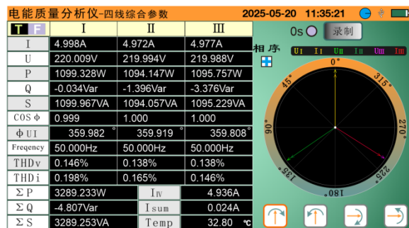
综合参数-三相四线测试界面
